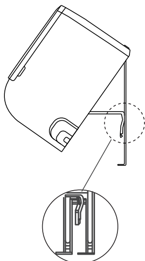
Na podoprenie jednotky použite držiak na zadnej strane jednotky proti montážnej doske
